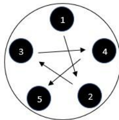
5 Lug Tightening
